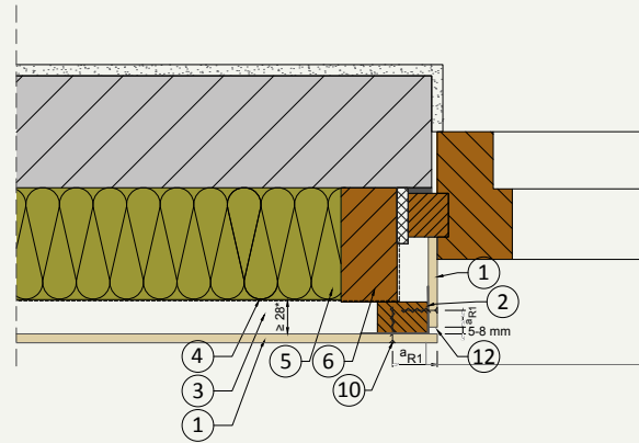
H.02 Vindusavslutning
