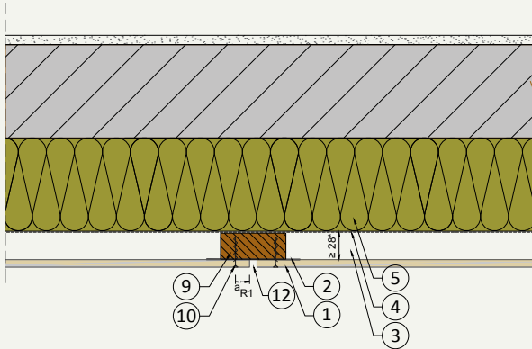
H.01 Vertikal skjøt
