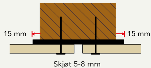
3. Bærende trekonstruksjon med vertikal skjøteløsning.
