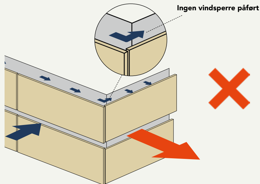
2. Mangel på vindspærre fører til problemer med vindbelastning
