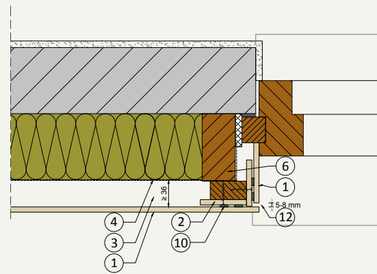
H.02 Vindusavslutning
