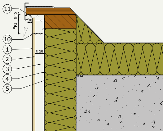
V.01 Gesims - parapet
