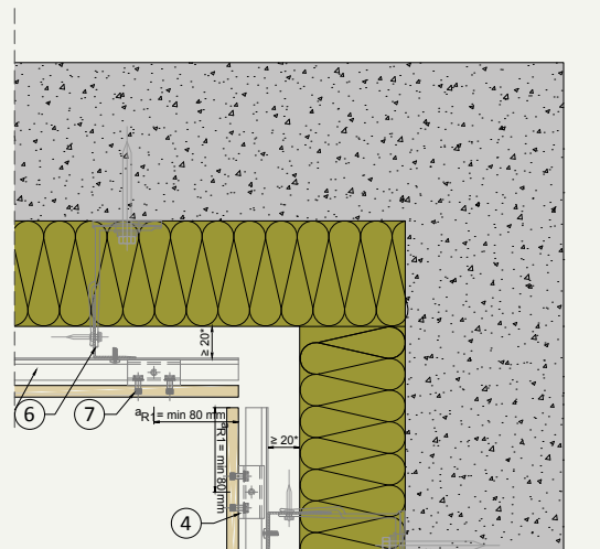
H.04 Innvendig hjørne
