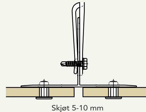
4. Bærende konstruksjon i aluminium/stål med vertikal skjøteløsning.
