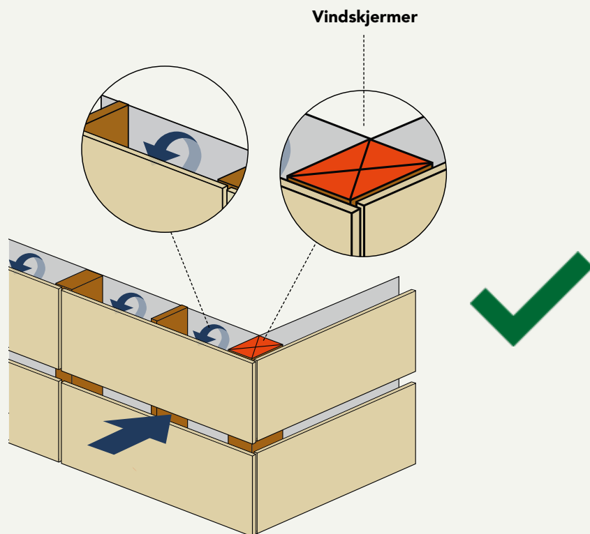
1. Vindspærren er korrekt påført
