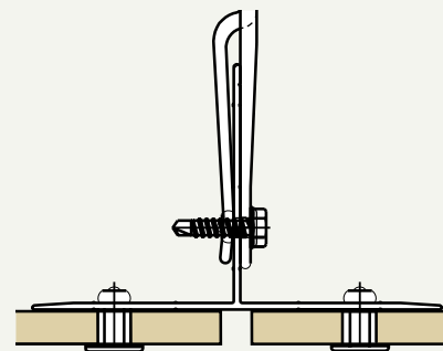
5. Løsning for vertikale skjøter i underkonstruksjoner av aluminium eller stål
