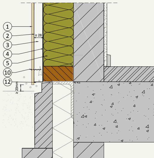
V.02 Avslutning mot terreng
