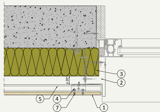
H.02 Vindusavslutning
