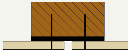
4. Underkonstruksjon av tre, vertikal fugeløsning med EPDM-tape.
