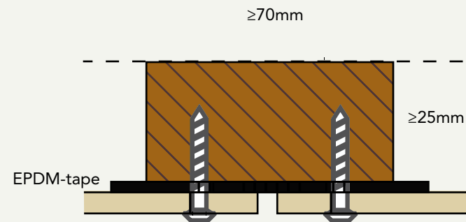
2. Innfesting i lekter (min. 70x25 mm) bak en skjøl
